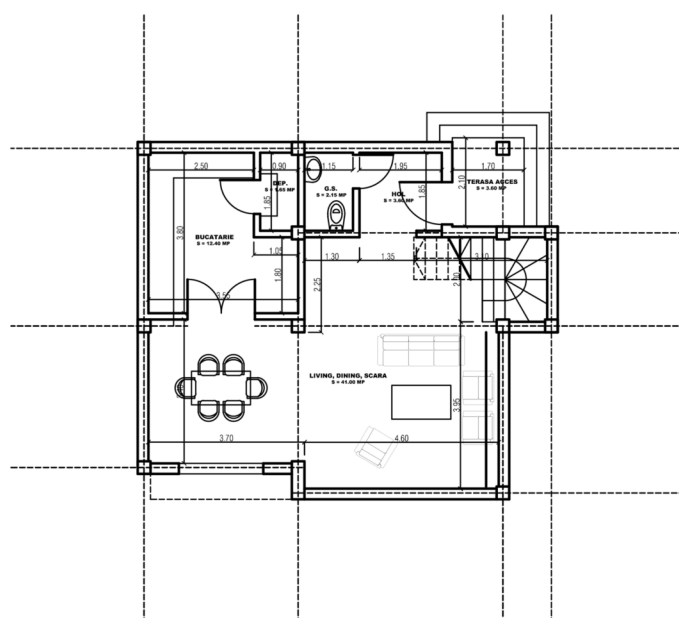
PLAN PARTER Suprafata construita: 72.35 mp Suprafata utila: 60.80 mp Suprafata terase: 3.60 mp Suprafata construita desfasurata: 148.55 mp Suprafata utila desfasurata: 119.55 mp Suprafata construita totala: 155.70 mp
