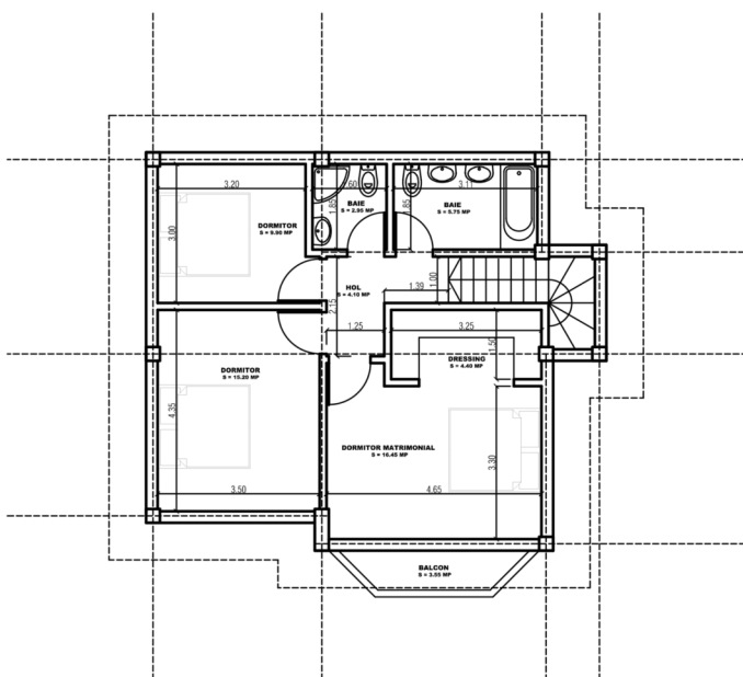
PLAN ETAJ Suprafata construita: 76.20 mp Suprafata utila: 58.75 mp Suprafata balcon: 3.55 mp Suprafata construita desfasurata: 148.55 mp Suprafata utila desfasurata: 119.55 mp Suprafata construita totala: 155.70 mp
